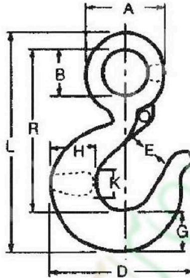
Gancho para cable Vulkan® S-320
