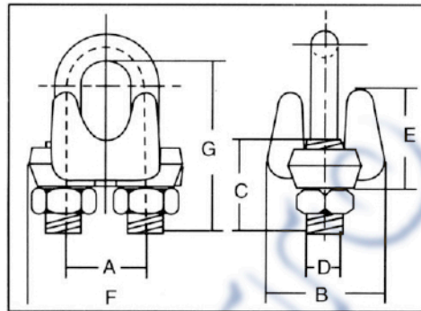
Grillete de acero forjado para cable Vulkan® G-450
