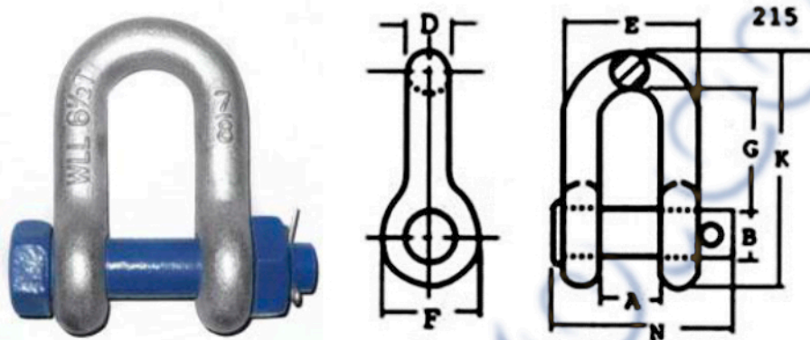
Grillete para carga tipo “U” Vulkan® G-2150
